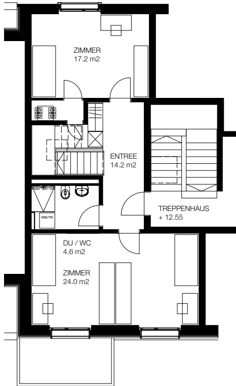
4. OBERGESCHOSS
