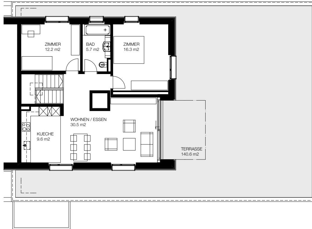
5. OBERGESCHOSS
