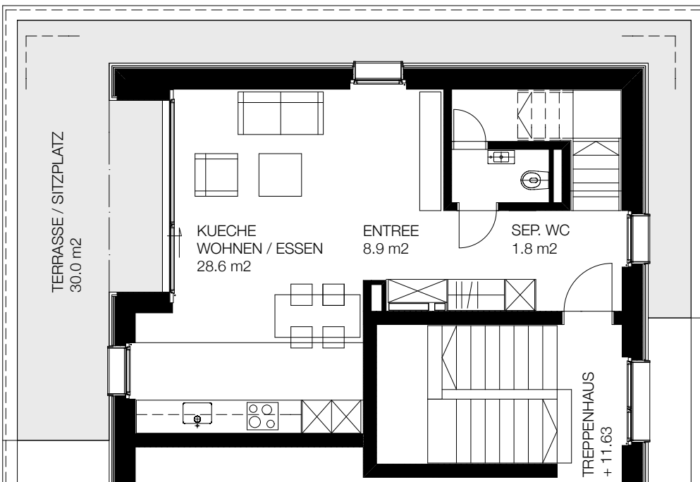
4. OBERGESCHOSS
