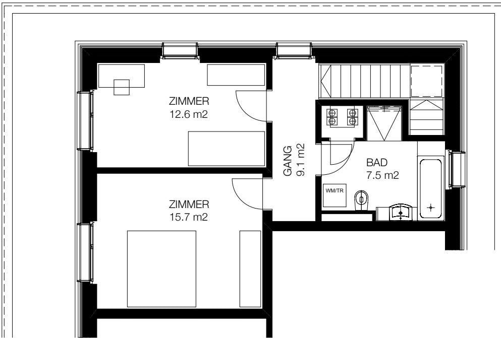
5. OBERGESCHOSS
