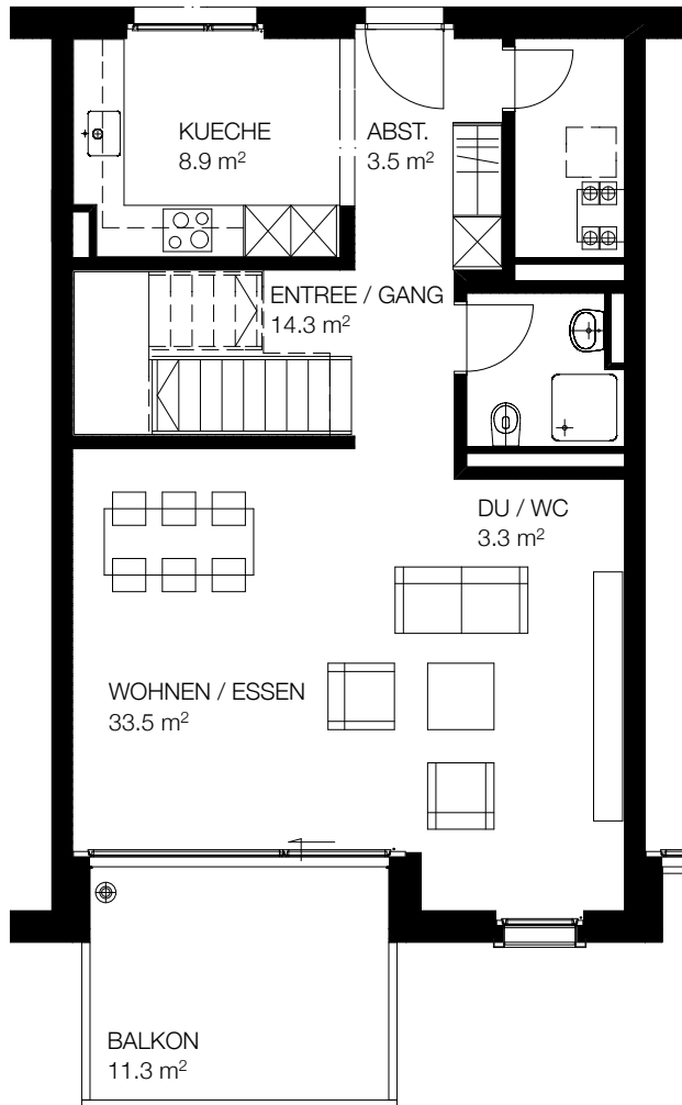
2. OBERGESCHOSS
