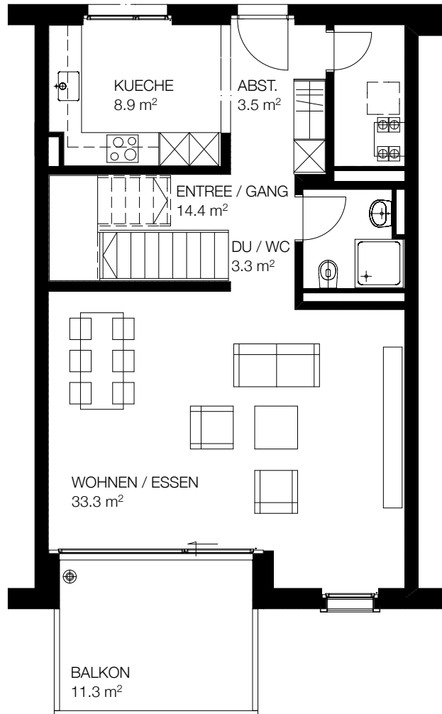
ERDGESCHOSS
